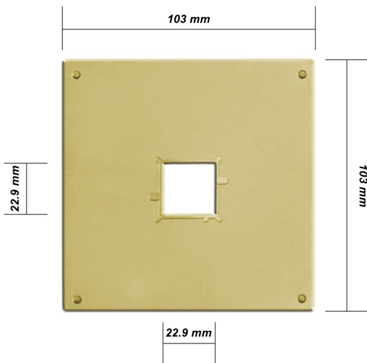
Aufbau Ansicht 01
