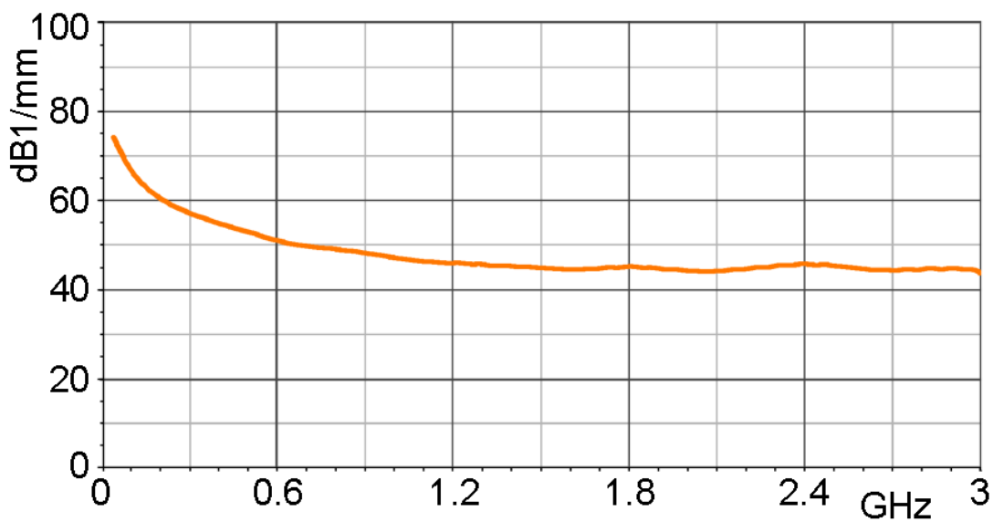
Korrekturkurve E-Feld [dBμV/mm] / [dBμV]
