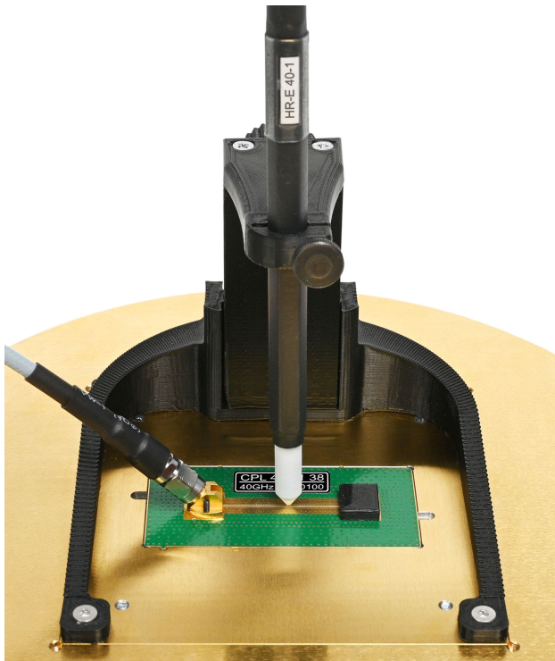
Messaufbau E-Feldsonde HR-E 40-1 auf 40 GHz Koplanarleitung
