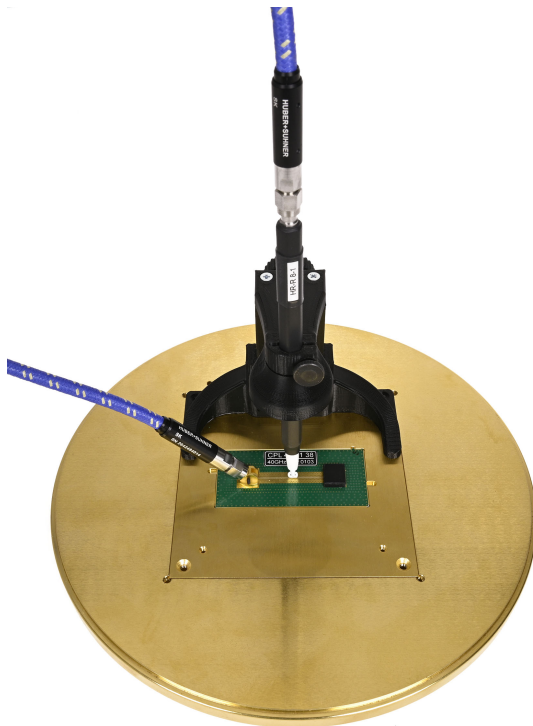
Messaufbau Magnetfeldsonde HR-R 8-1 auf 40 GHz Koplanarleitung
