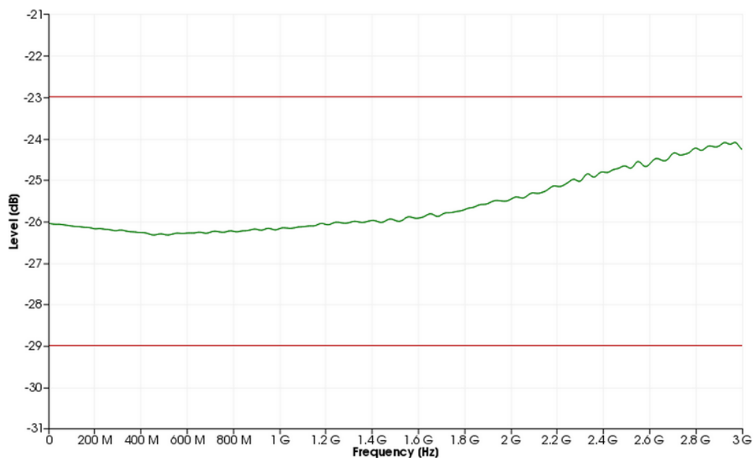
频率特性
