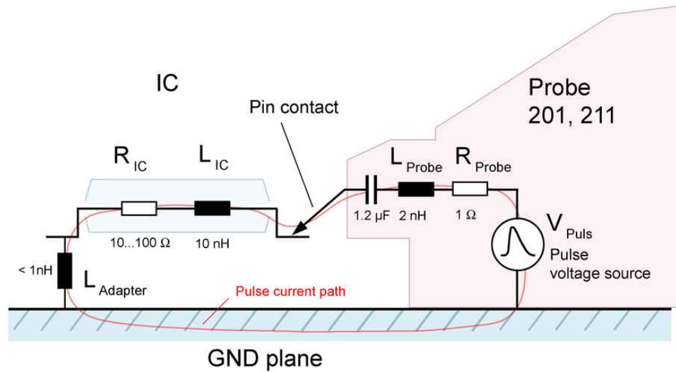
等效电路图
